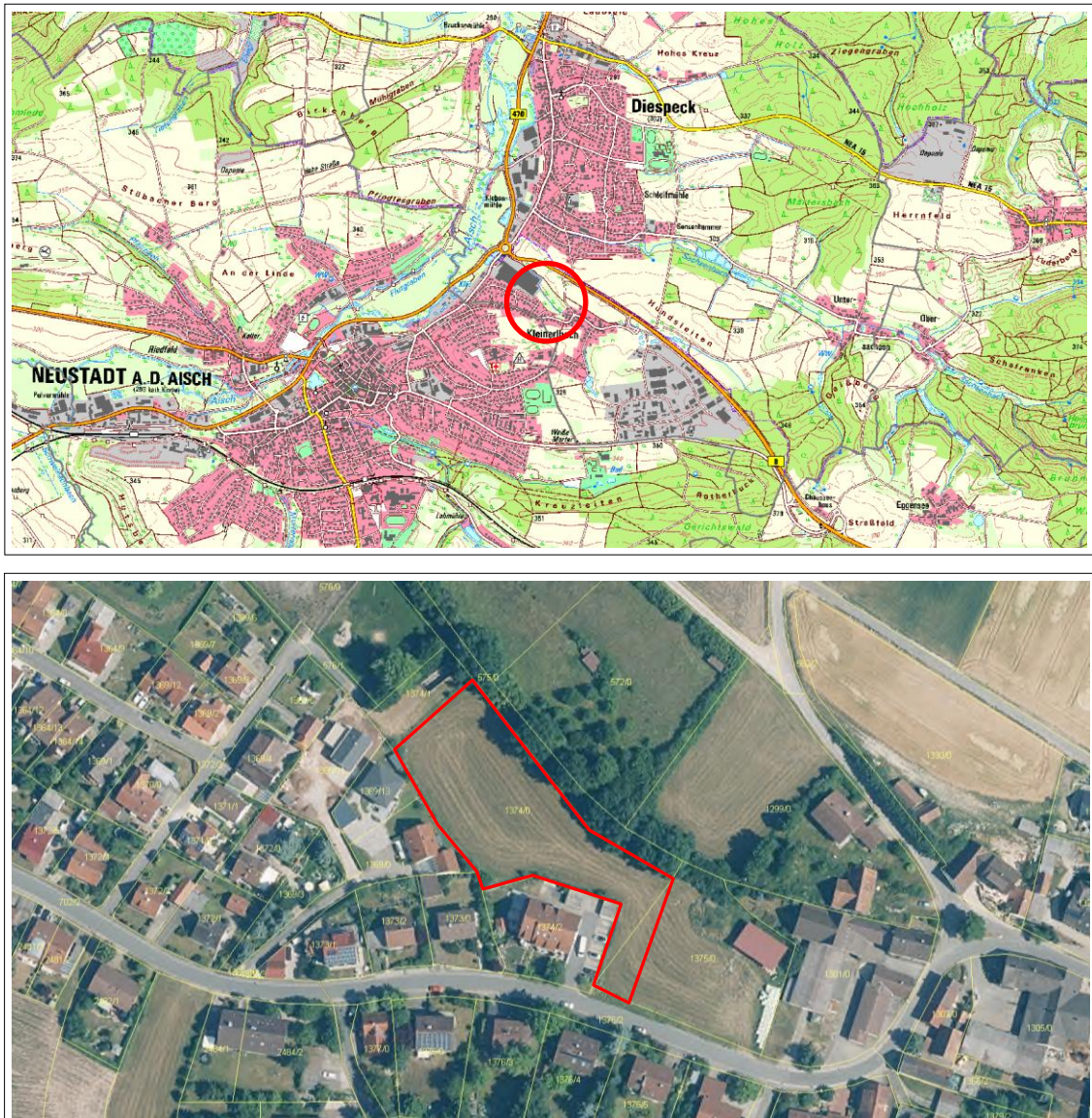
Abb. 1 und 2: Lage und Abgrenzung der Fläche für den Bau eines Regenrückhaltebeckens.
